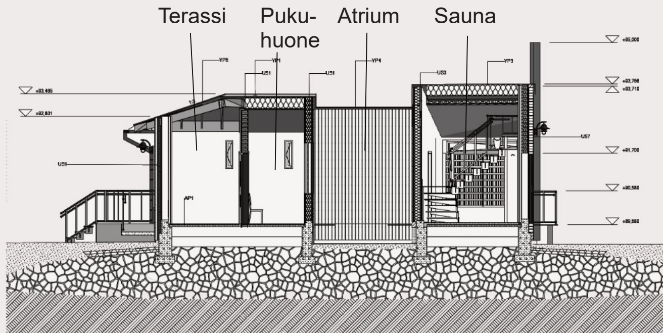
Leikkaus idästä
