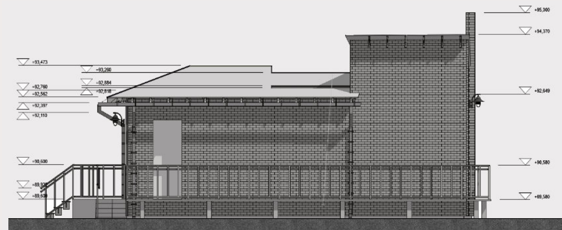
Julkisivu itään
